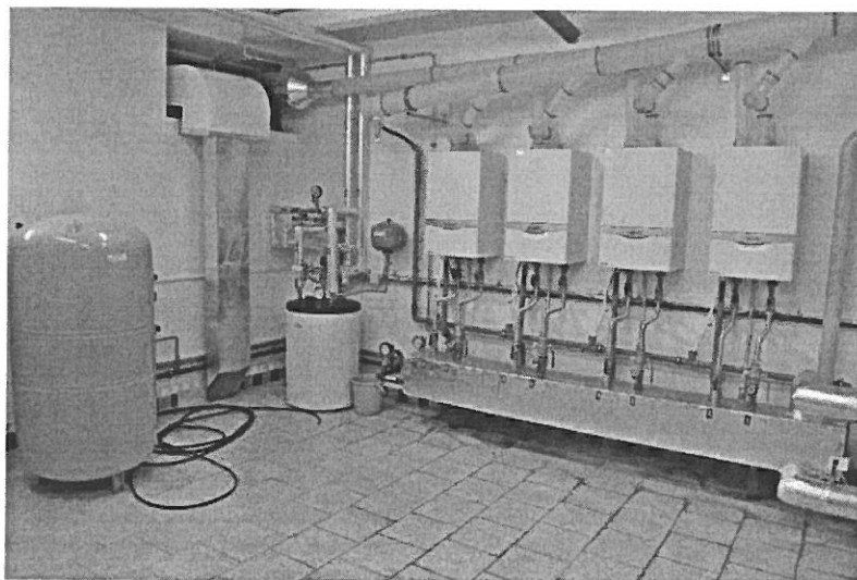
Rekonstrukce kotelny
